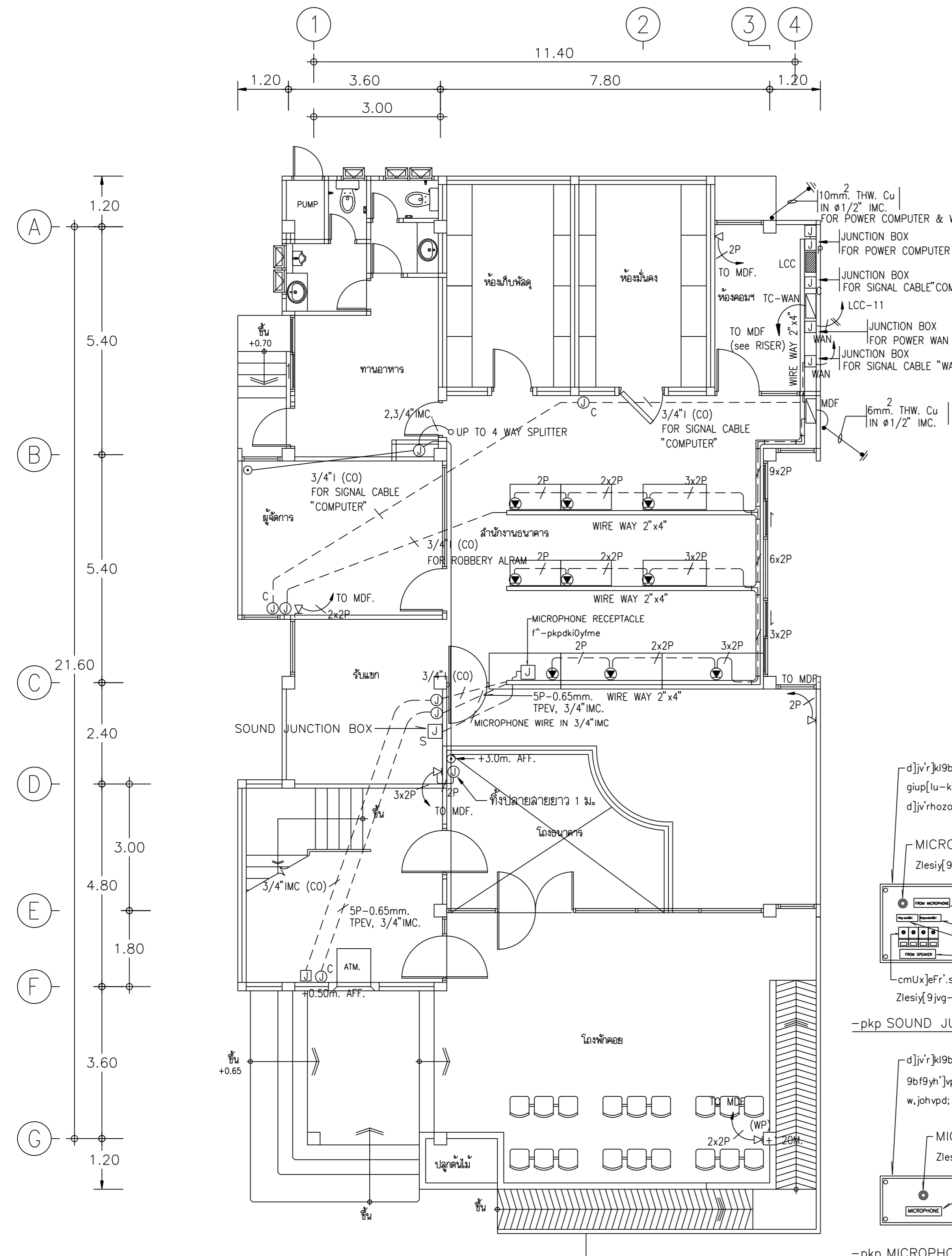
แปลนติดตั้งระบบเดำารโทรศัพท์ และโทรศัพท์ ชั้นล่าง
