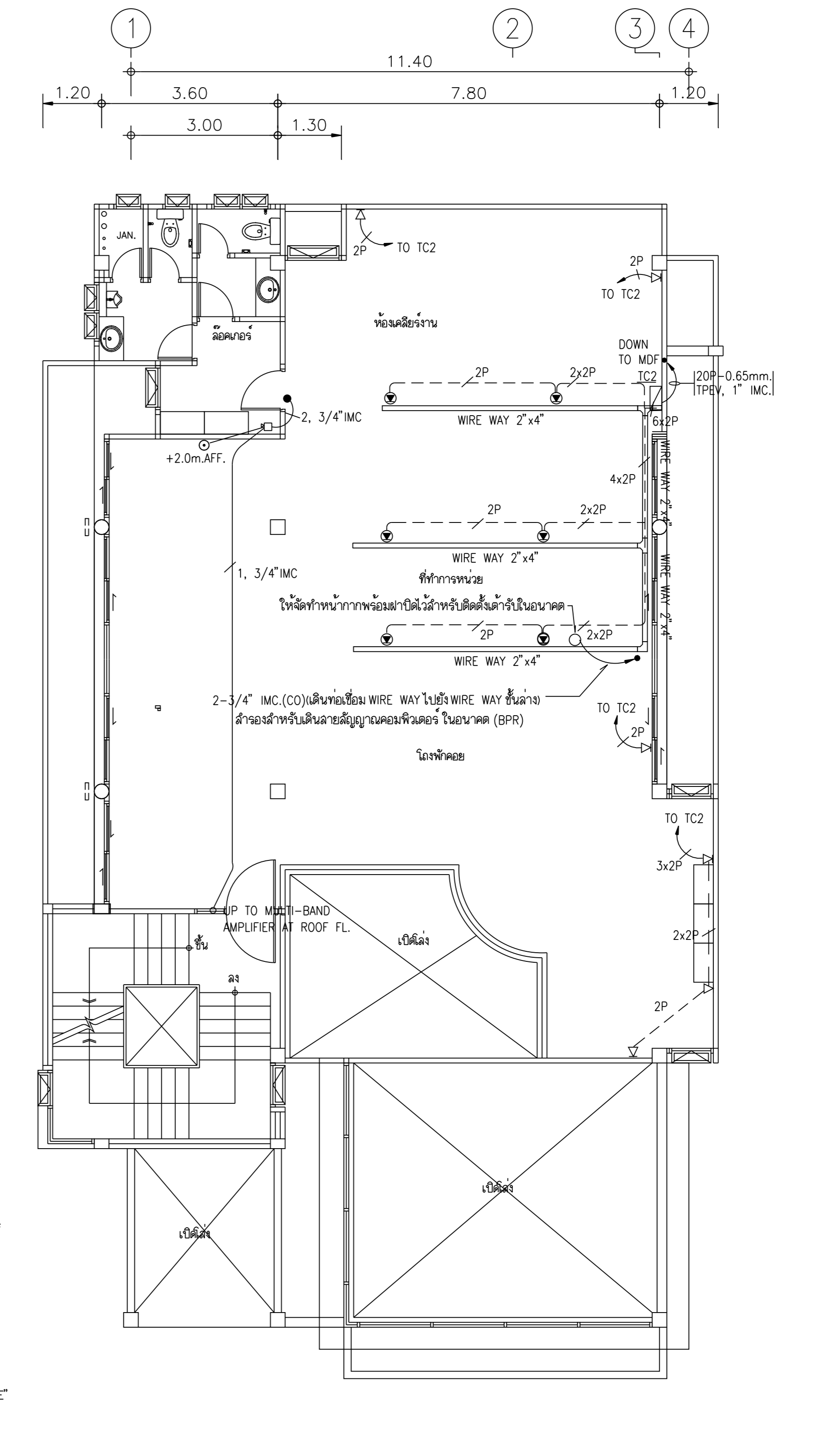
แปลนติดตั้งระบบเดำารโทรศัพท์ และโทรศัพท์ ชั้น 2
