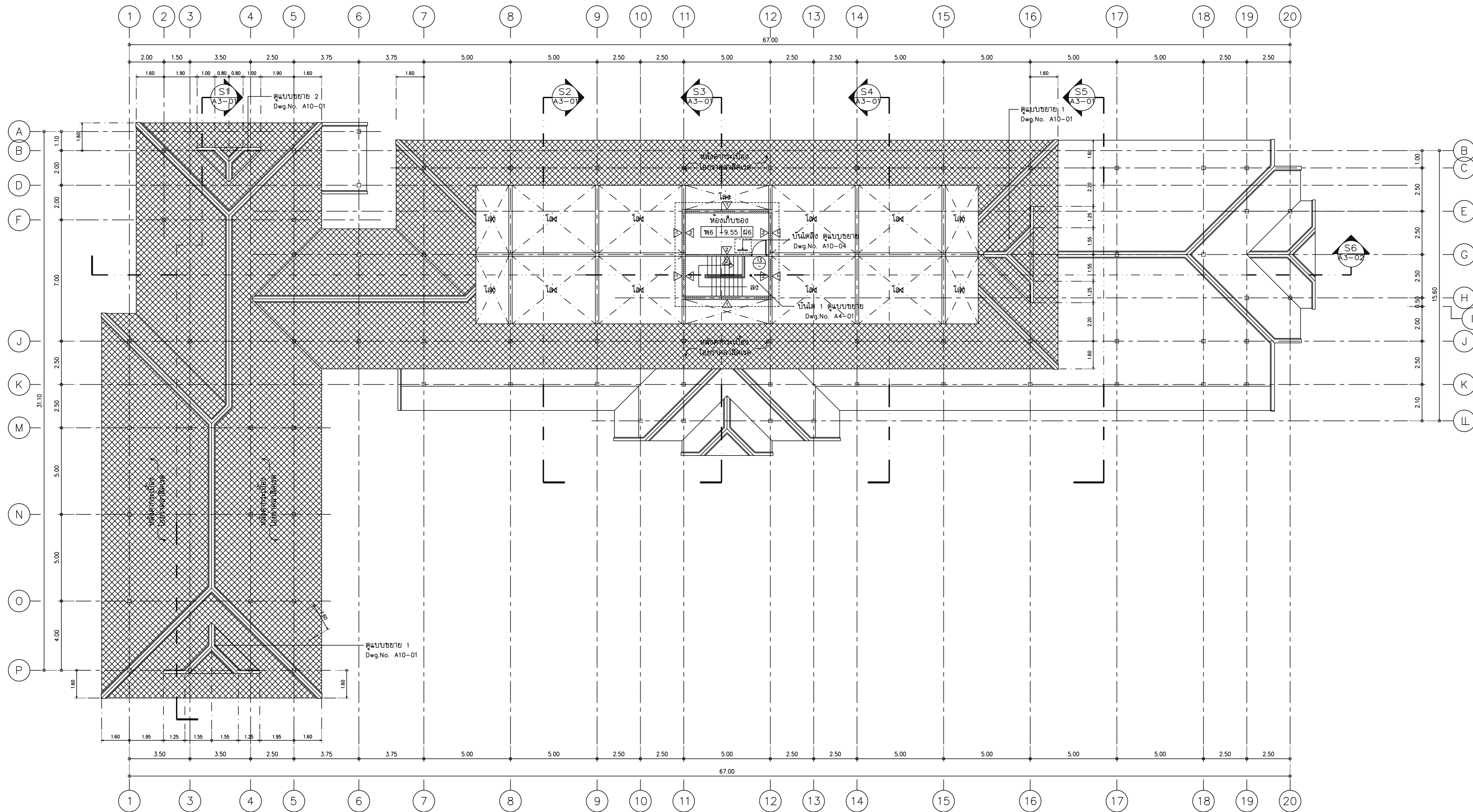
แปลนห้องเก็บของใต้หลังคา มาตราส่วน 1 : 125
