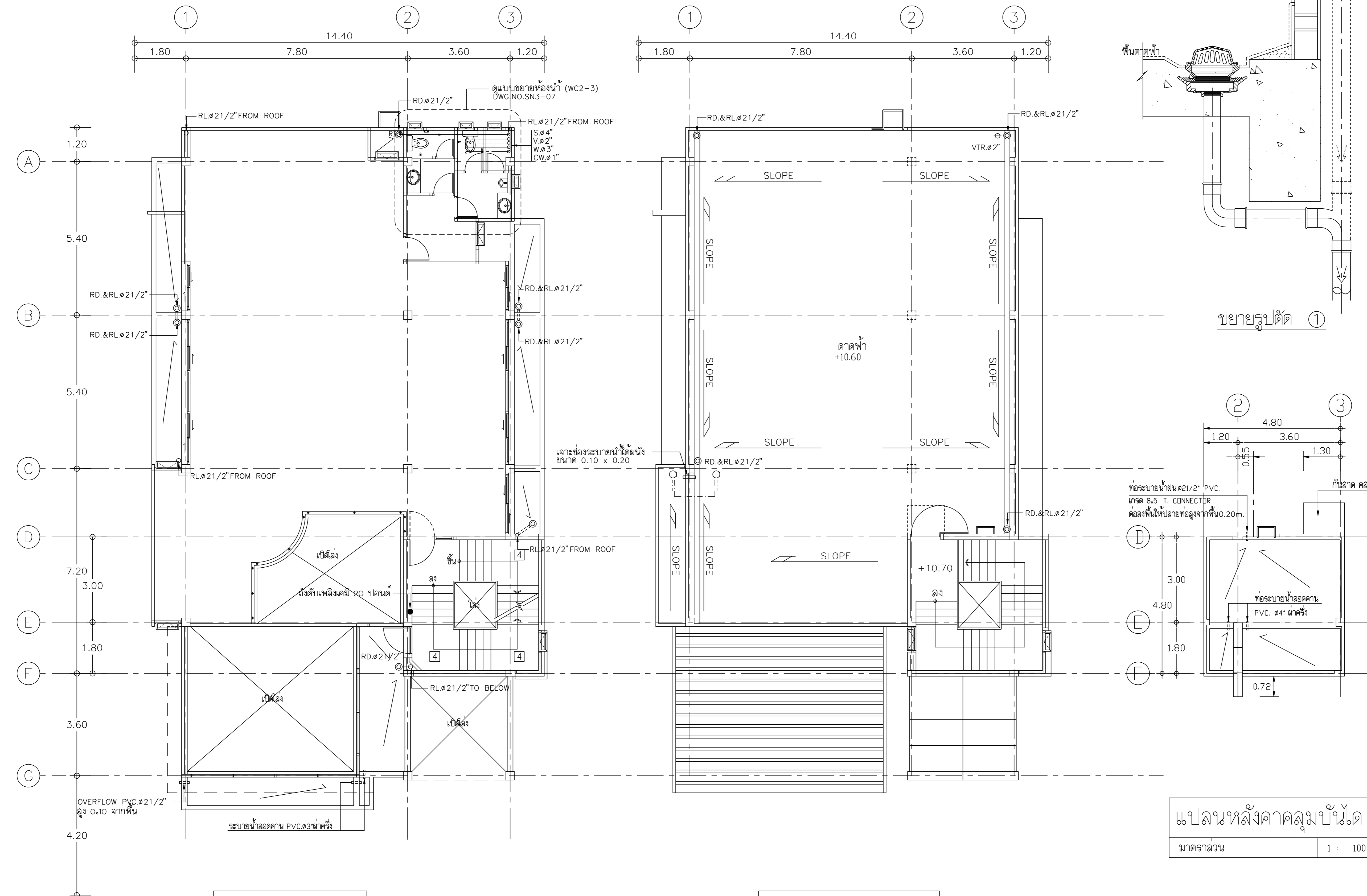
แปลนพื้นที่ชั้น 3 มาตราส่วน 1 : 100 หมายเหตุ แนวท่อดำงา ให้ดูแบบสถาปัตยกรรมและแบบโครงสร้างประกอบ
