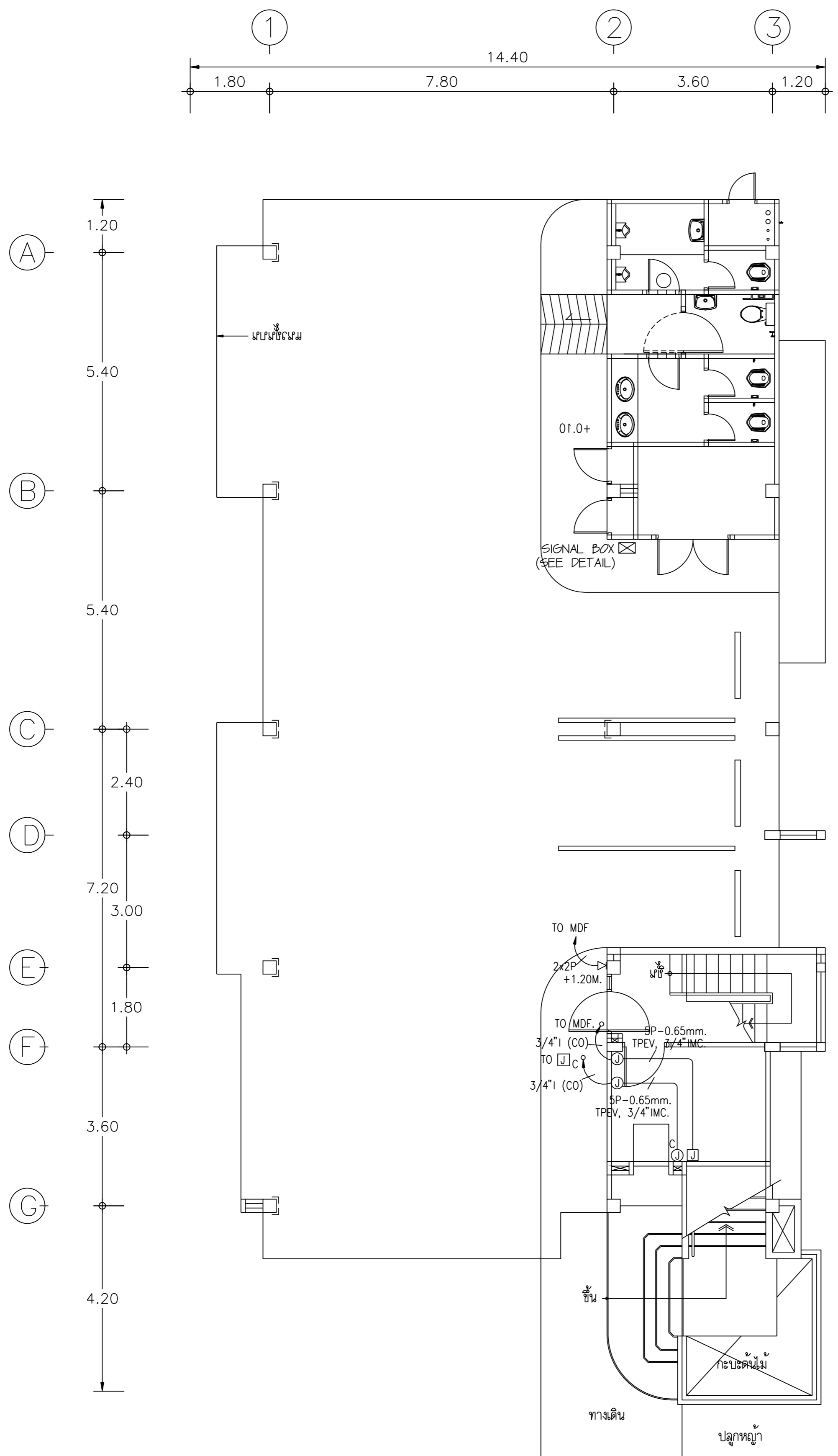
แปลนติดตั้งระบบเดำรับโทรศัพฑ์ ชั้นล่าง
