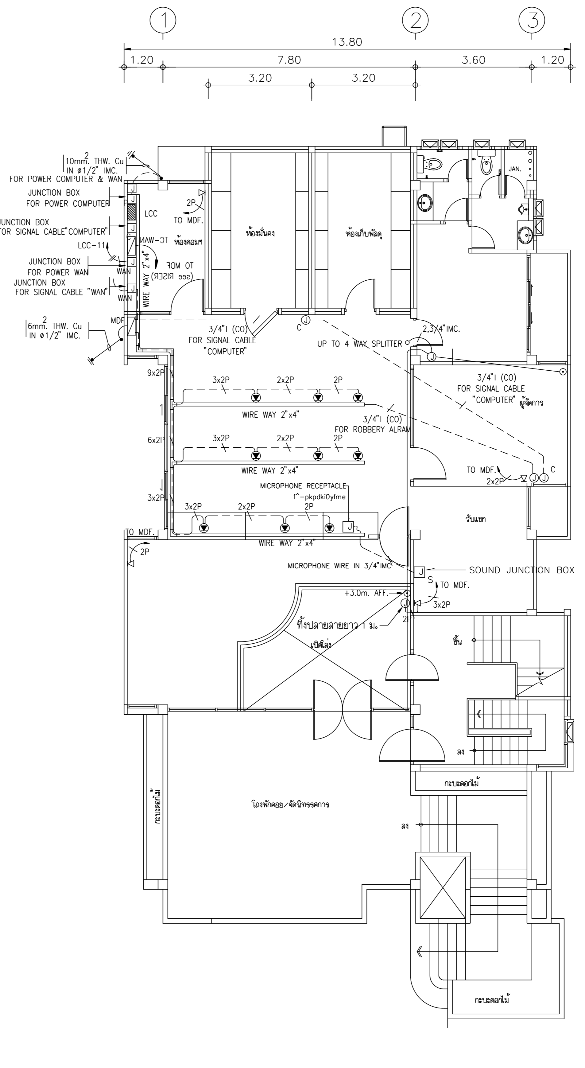
แปลนติดตั้งระบบเดำรับโทรศัพฑ์ และเดำรับลยอากาศโทรศัพฑ์ ชั้น.2
