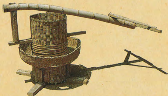
เครื่องสีข้าว ใช้สีหรือขัดข้าวเปลือกให้เป็นข้าวสาร
