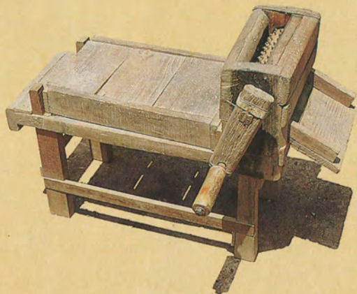
เครื่องตีข้าวโพด ใช้ตีเมล็ดข้าวโพดออกจากฝัก
