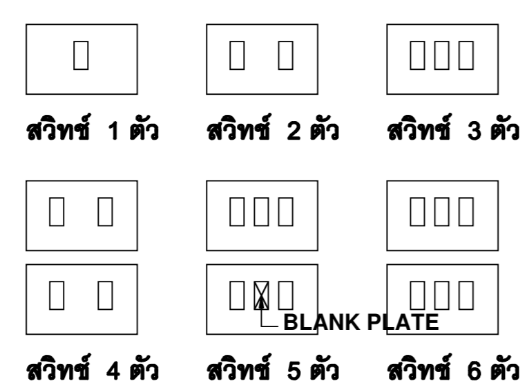
แบบแสดงการติดตั้งสวิทช์
