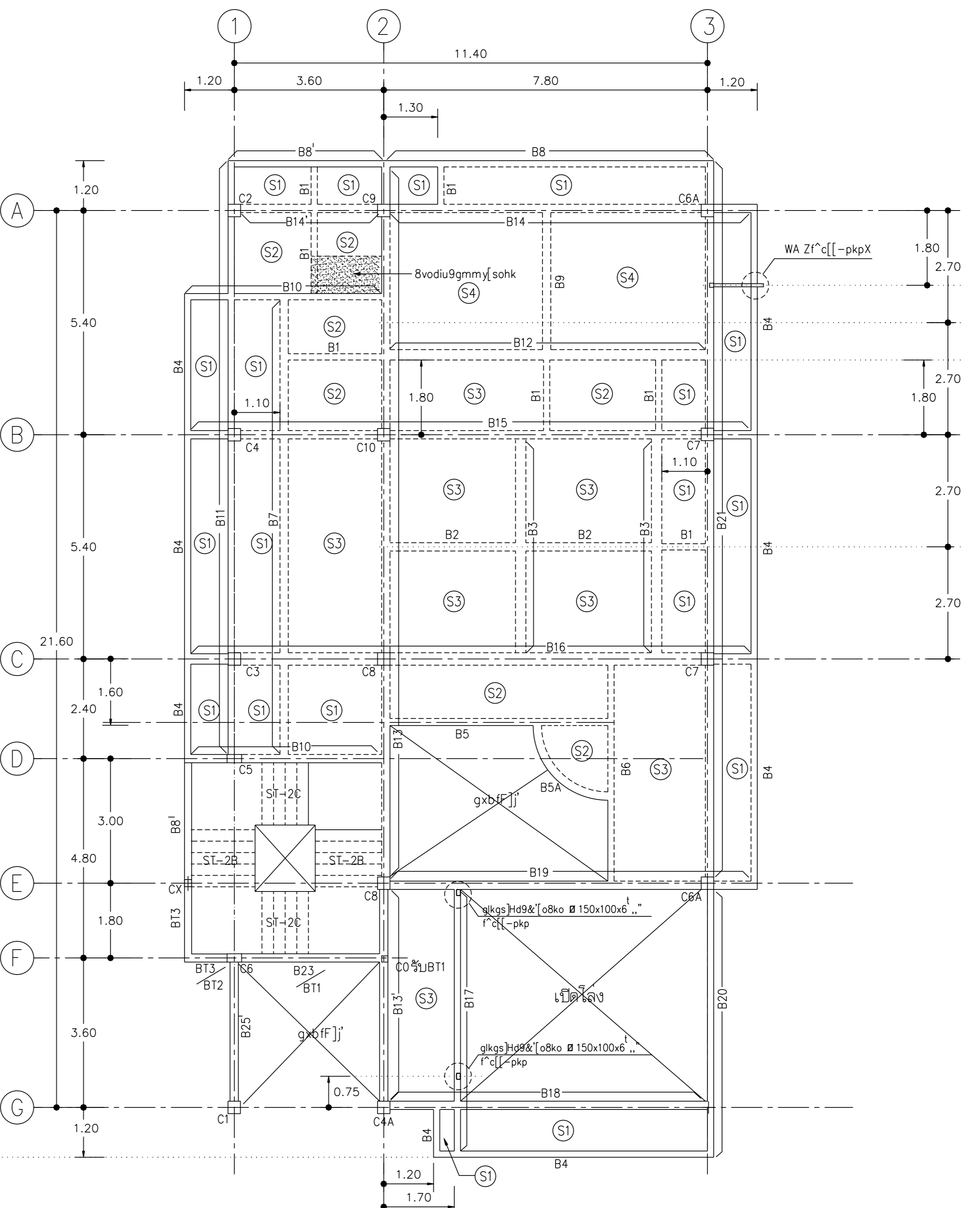
แปลนเสาคานและพื้นชั้น 3 มาตราส่วน 1 : 100
