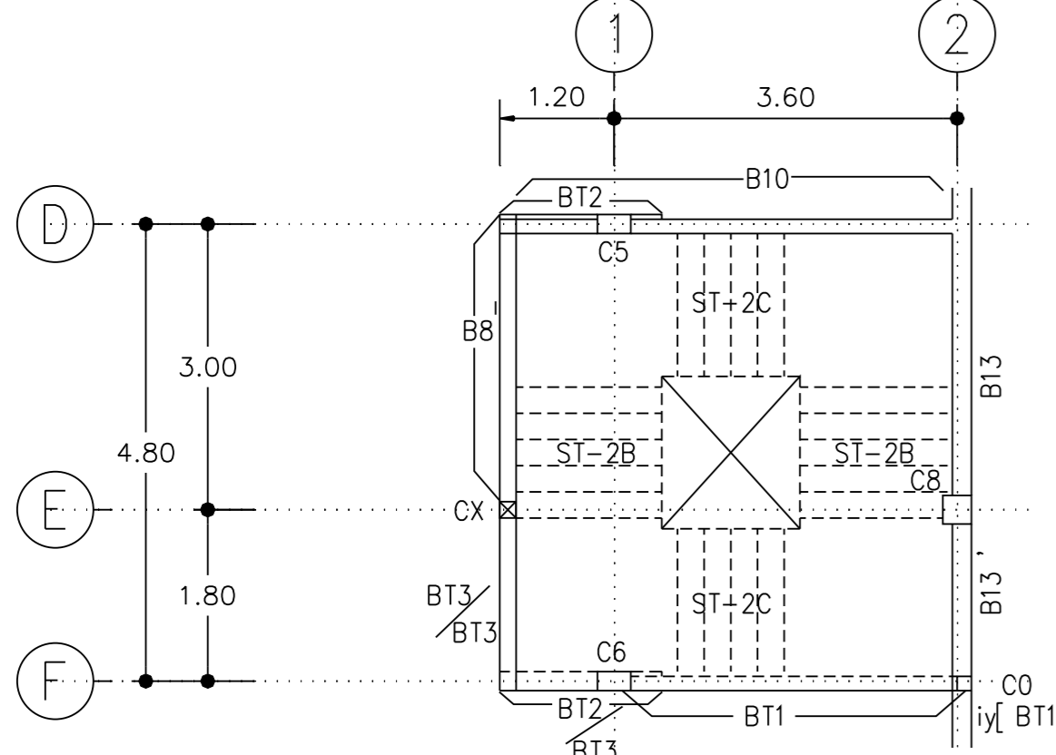
แปลนเสาคานและพื้นชั้น 2 มาตราส่วน 1 : 100
