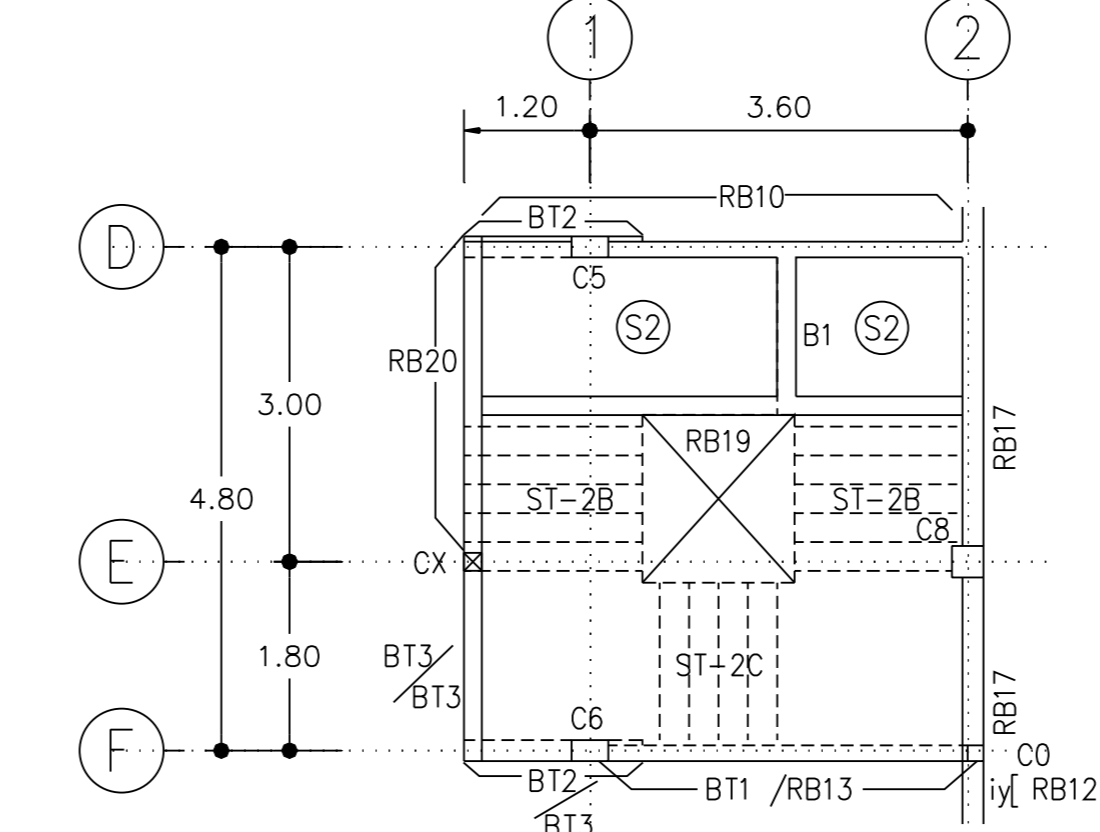
แปลนเสาคานและพื้นชั้น 3 มาตราส่วน 1 : 100
