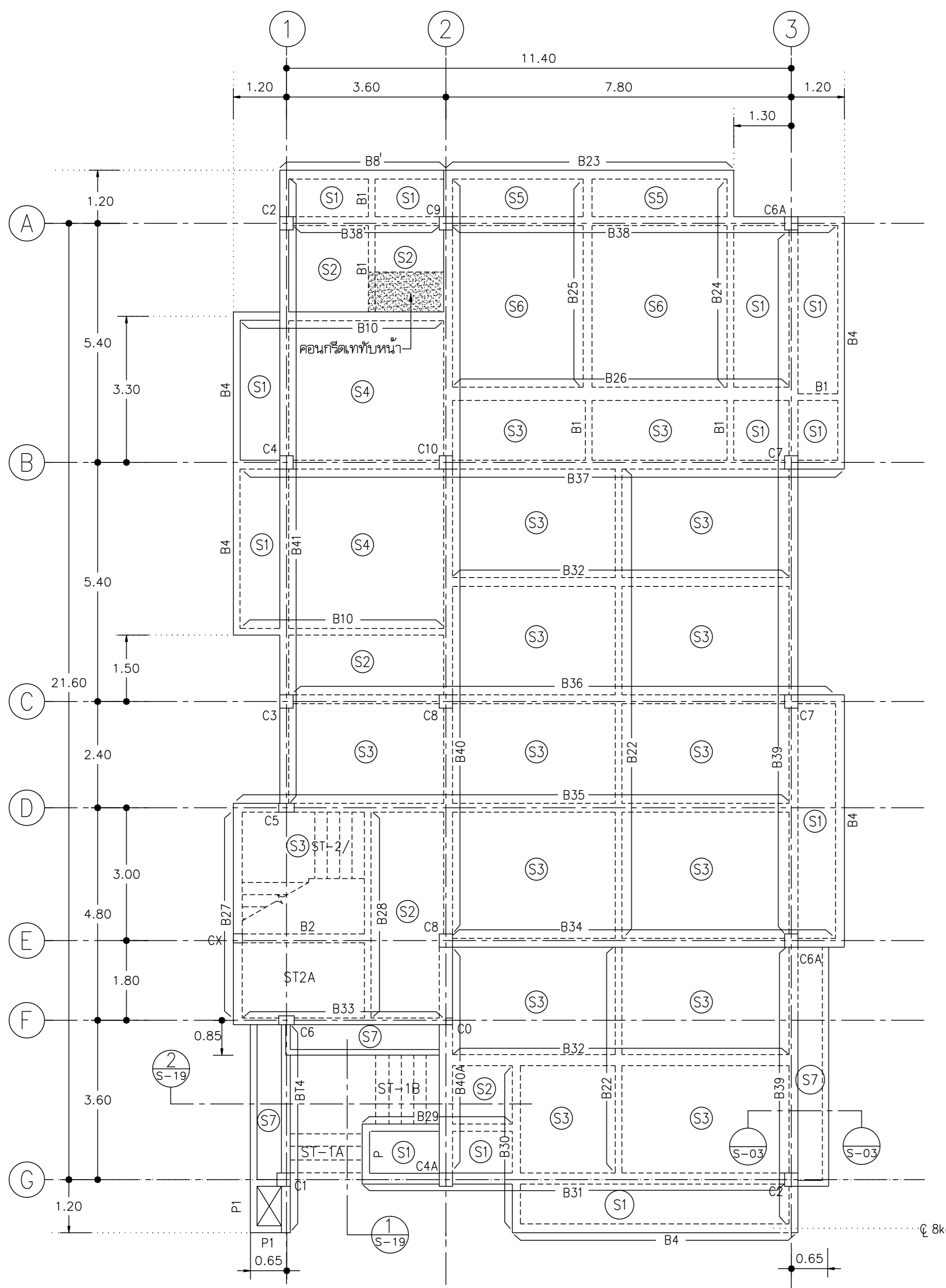
แปลนเสาคานและพื้นชั้น 2 มาตราส่วน 1 : 100
