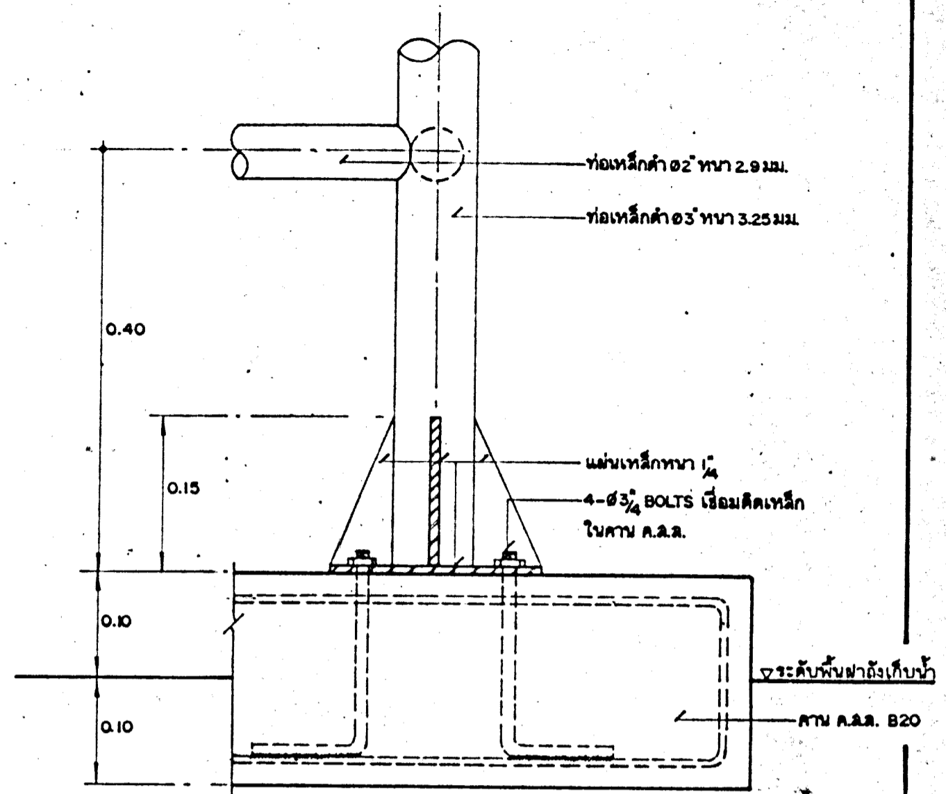
แบบขยาย 1 1:85
