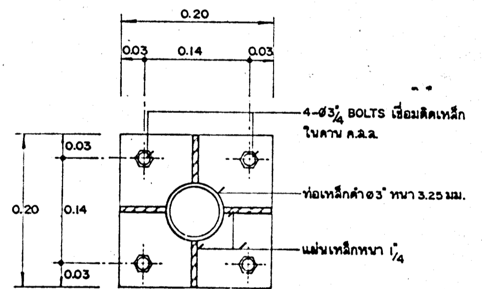
แบบขยายแผ่นเหล็ก 1:85
