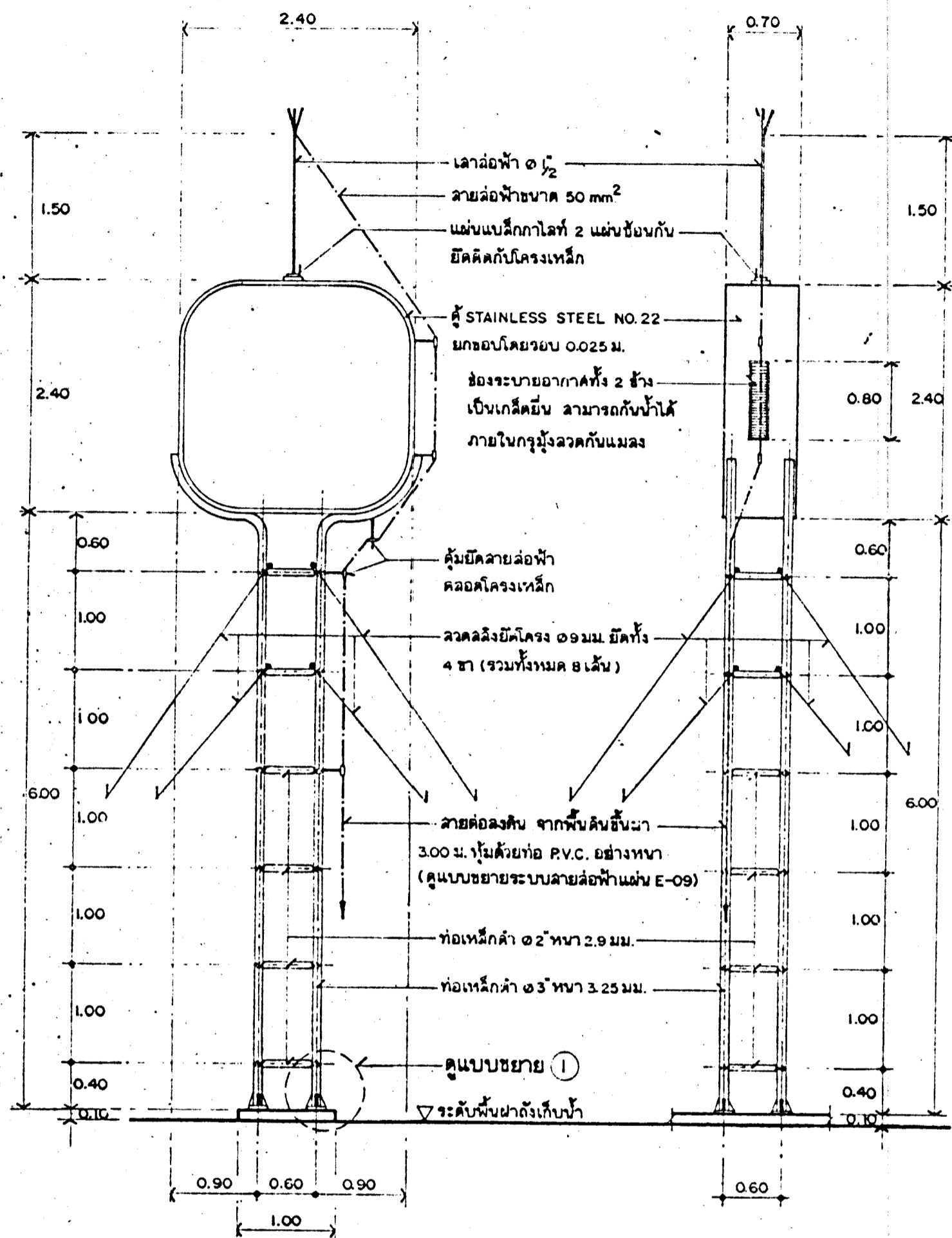
รูปด้านหน้า 1:50
