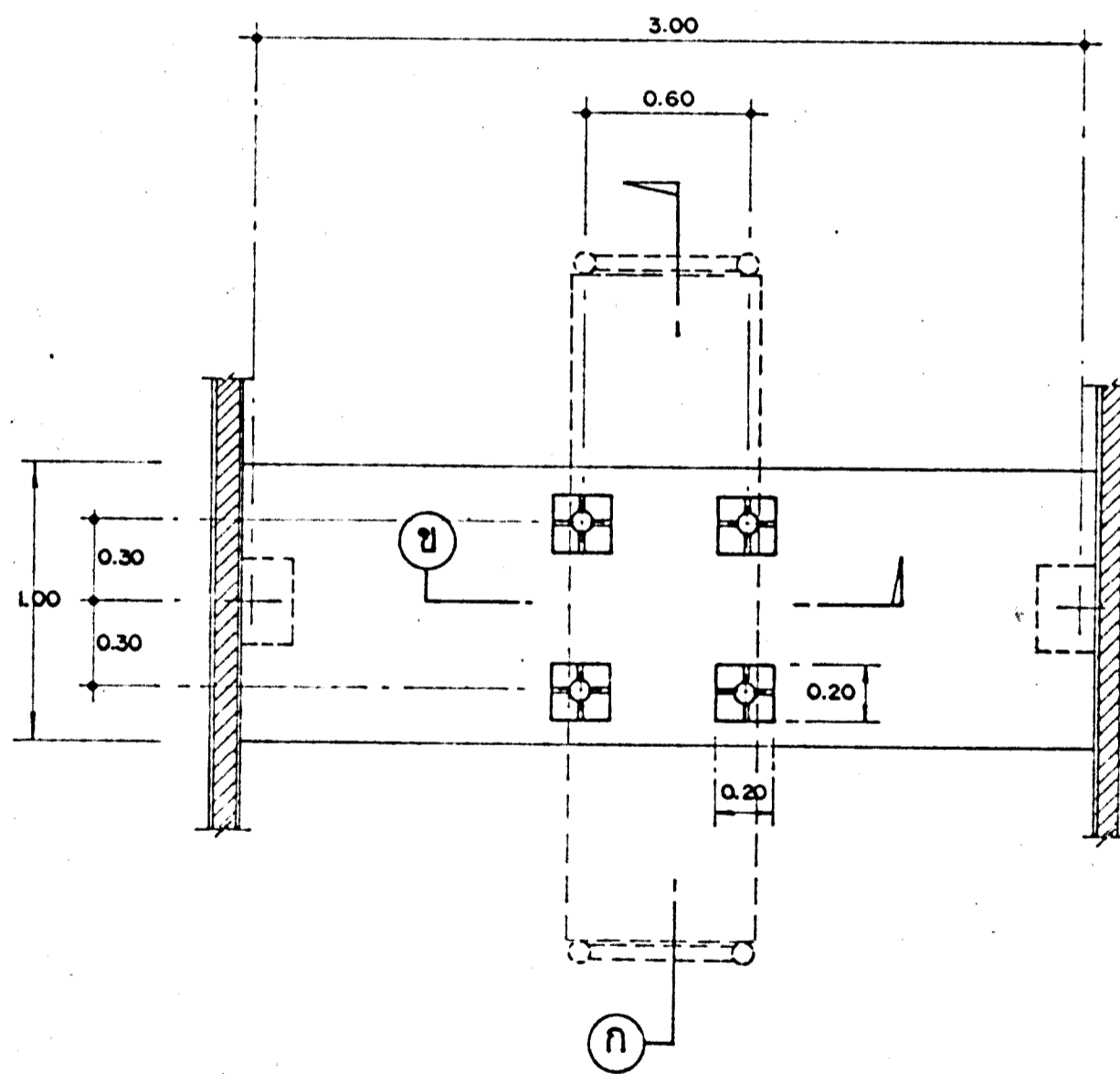
แปลนโลโก้ 1:25
