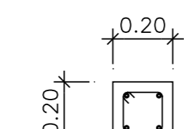
รูปตัด 1 - 1 1:25 ขนาด 0.20x0.20 เหล็กเสริม 4-DB12mm. เหล็กปลอก ๑6mm.๑0.20m.
