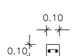
ขยายเสาเอ็น คสล. 1:25 ขนาด 0.10x0.10 เหล็กเสริม 2-๑9mm. เหล็กปลอก ๑6mm.๑0.20m.
