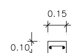
ขยายเสาเอ็น คสล. 1:25 ขนาด 0.10x0.15 เหล็กเสริม 2-๑9mm. เหล็กปลอก ๑6mm.๑0.20m.
