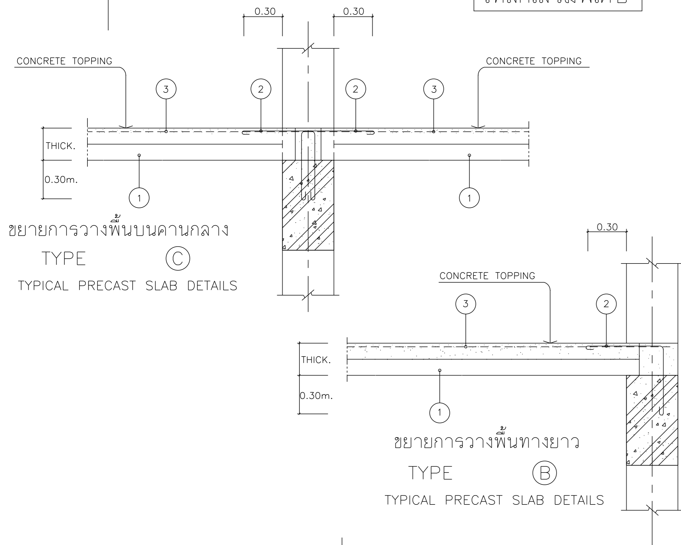
ขยายการวางพื้นทางขวาง TYPE (A) TYPICAL PRECAST SLAB DETAILS
