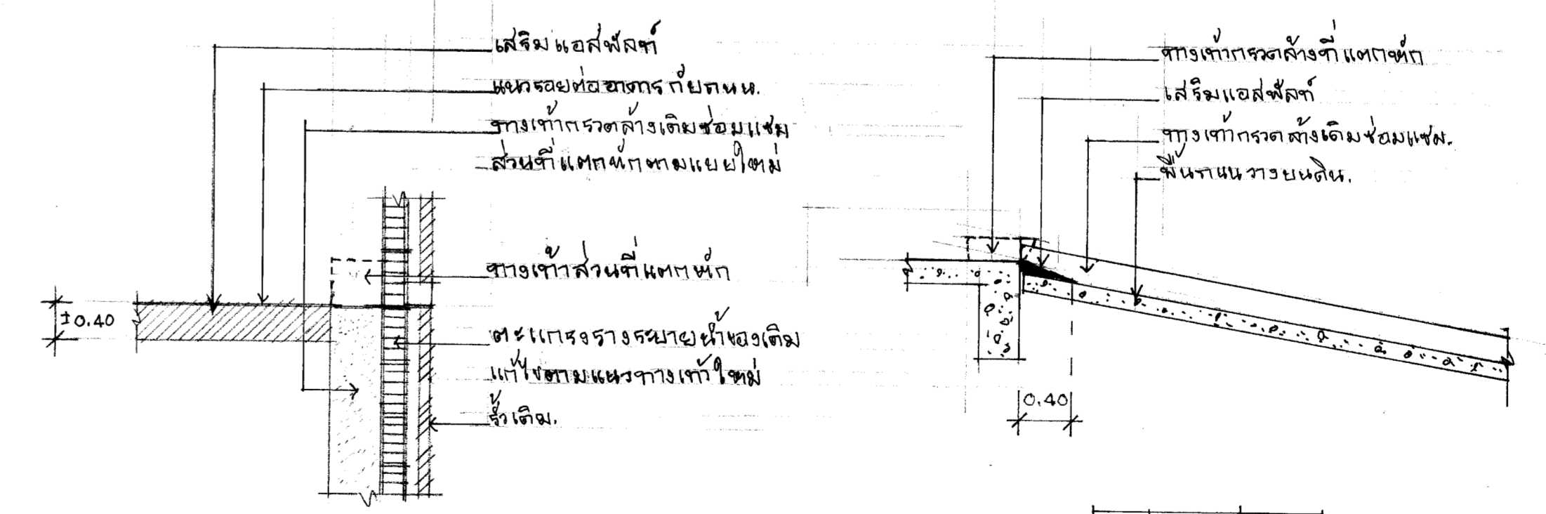
รูปตัดตามแนวยาย 1:50
