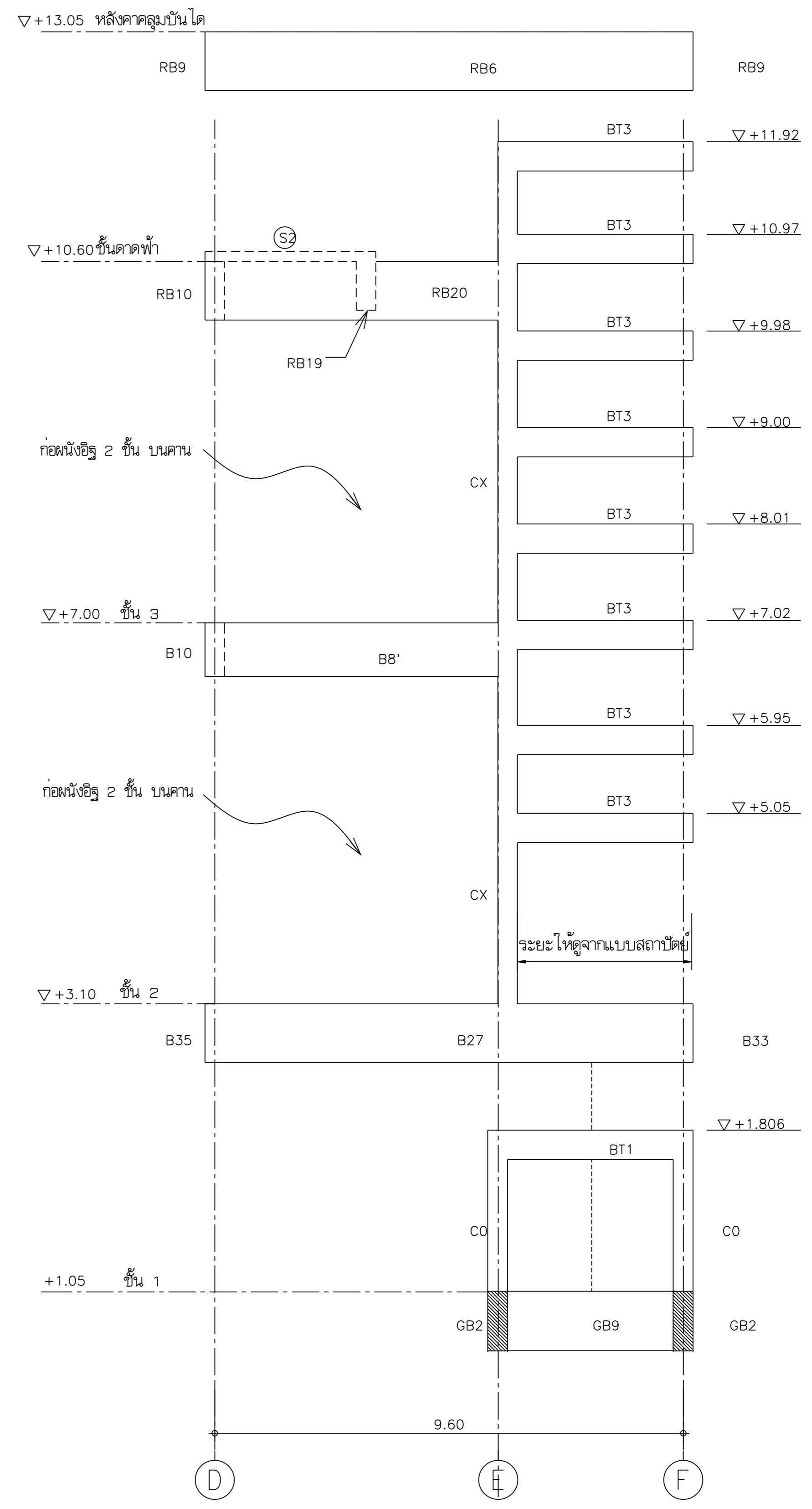
รูปด้านหลังบันได ST2 มาตราส่วน 1 : 50
