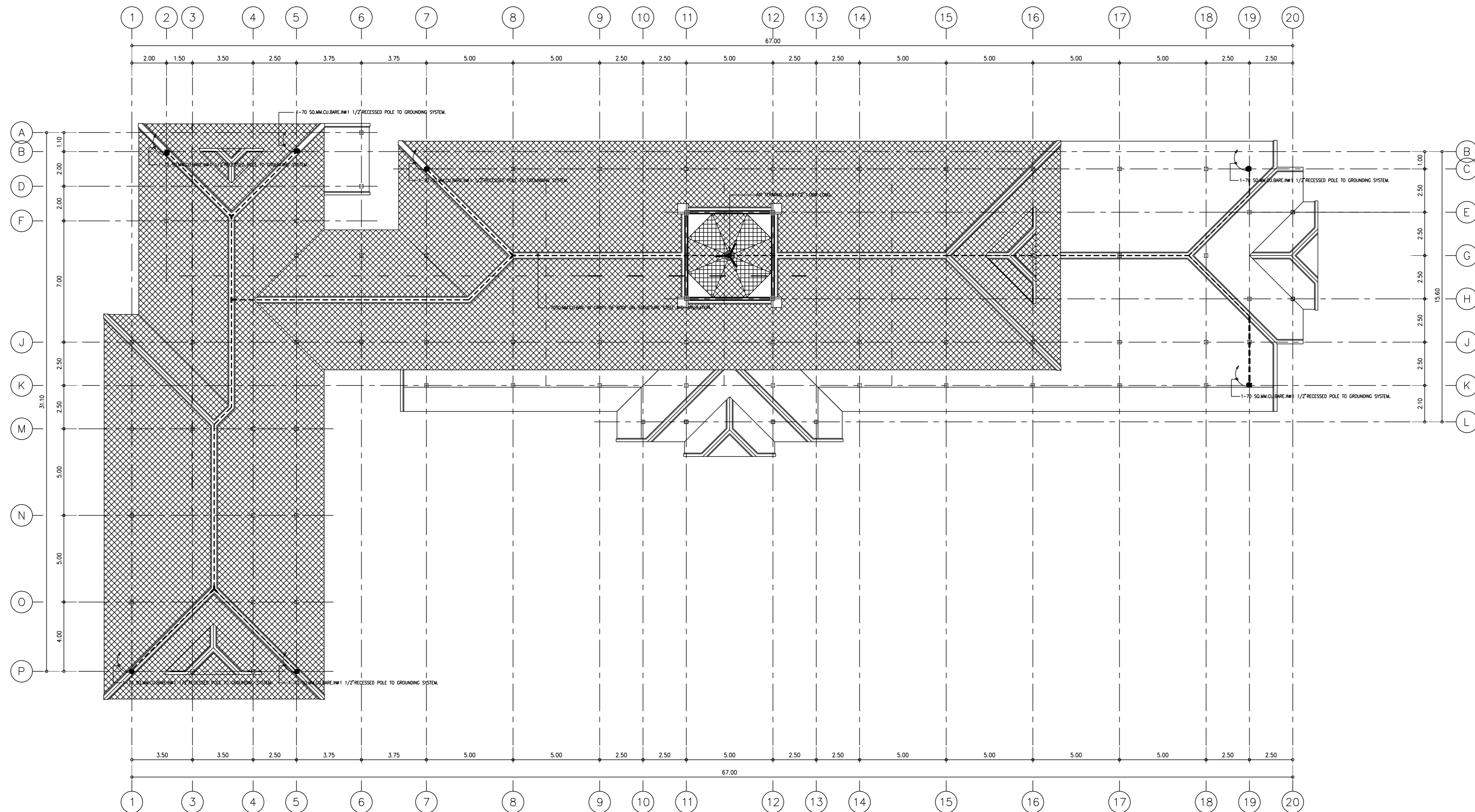
AIR TERMINAL & LIGHTNING ARRESTER WIRING. มาตรฐาน 1 : 125
