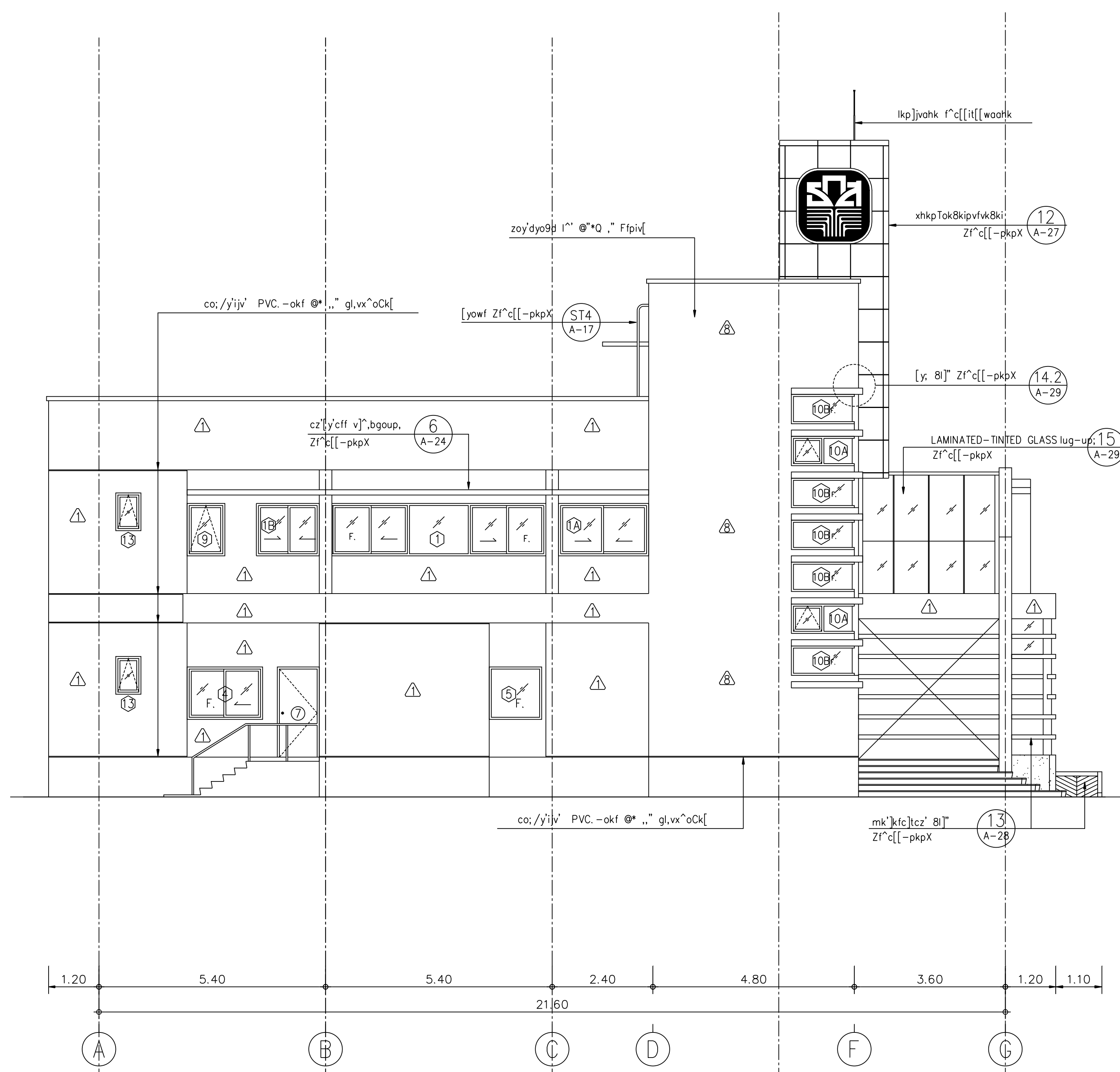
i^xfhko 2 k9ikl;o 1 : 100
