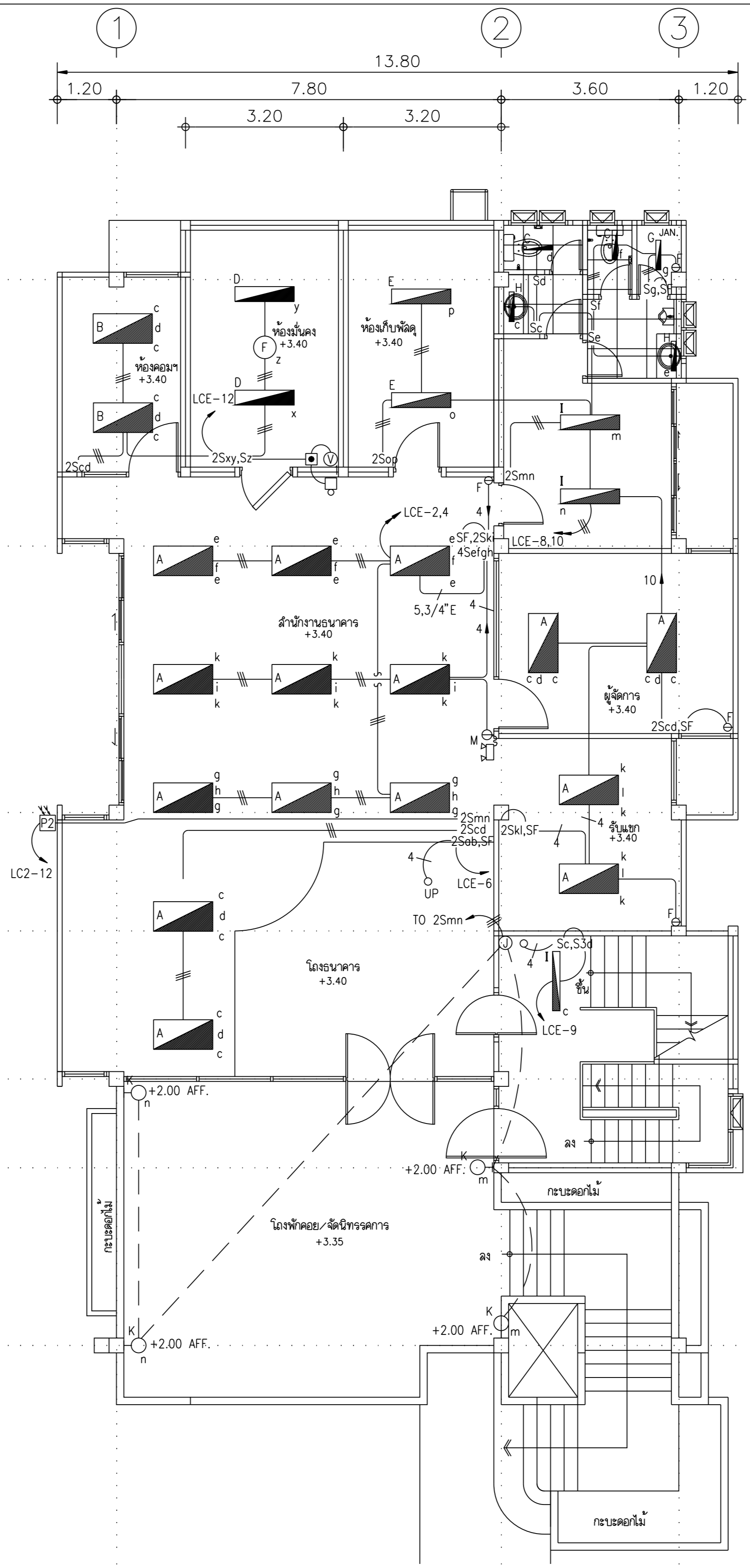
แปลนพื้นที่ชั้น 2 มาตราส่วน 1 : 100
