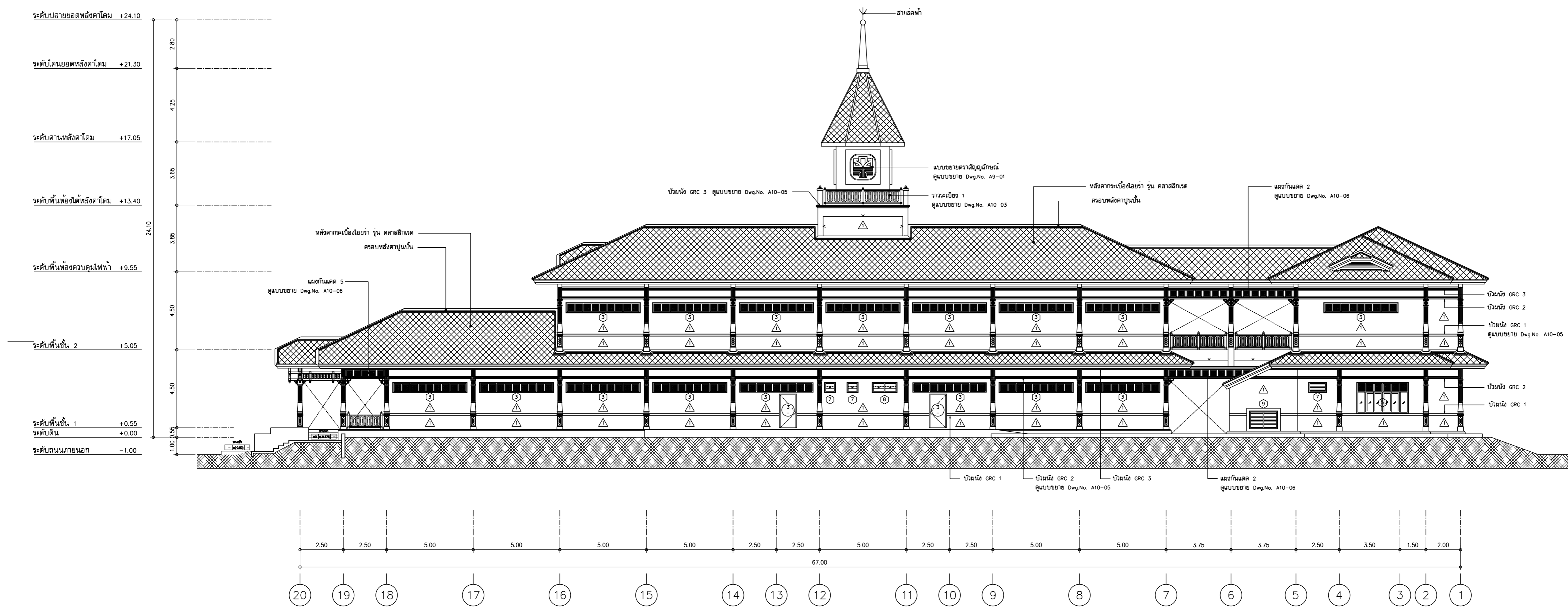
รูปด้าน C ขนาดส่วน 1 : 125
