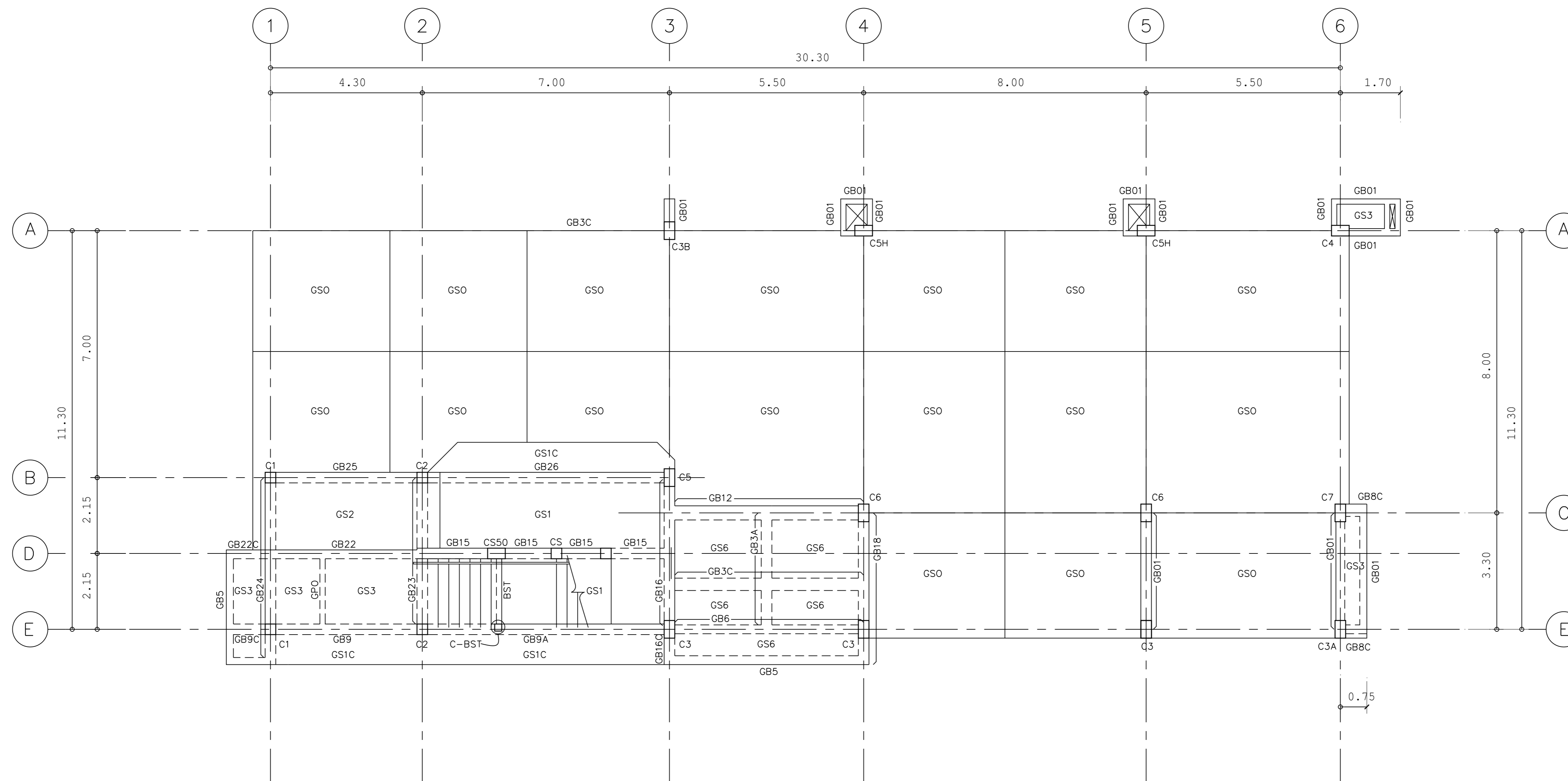
แปลนคานพื้นชั้นล่าง มาตรฐาน 1 : 100
