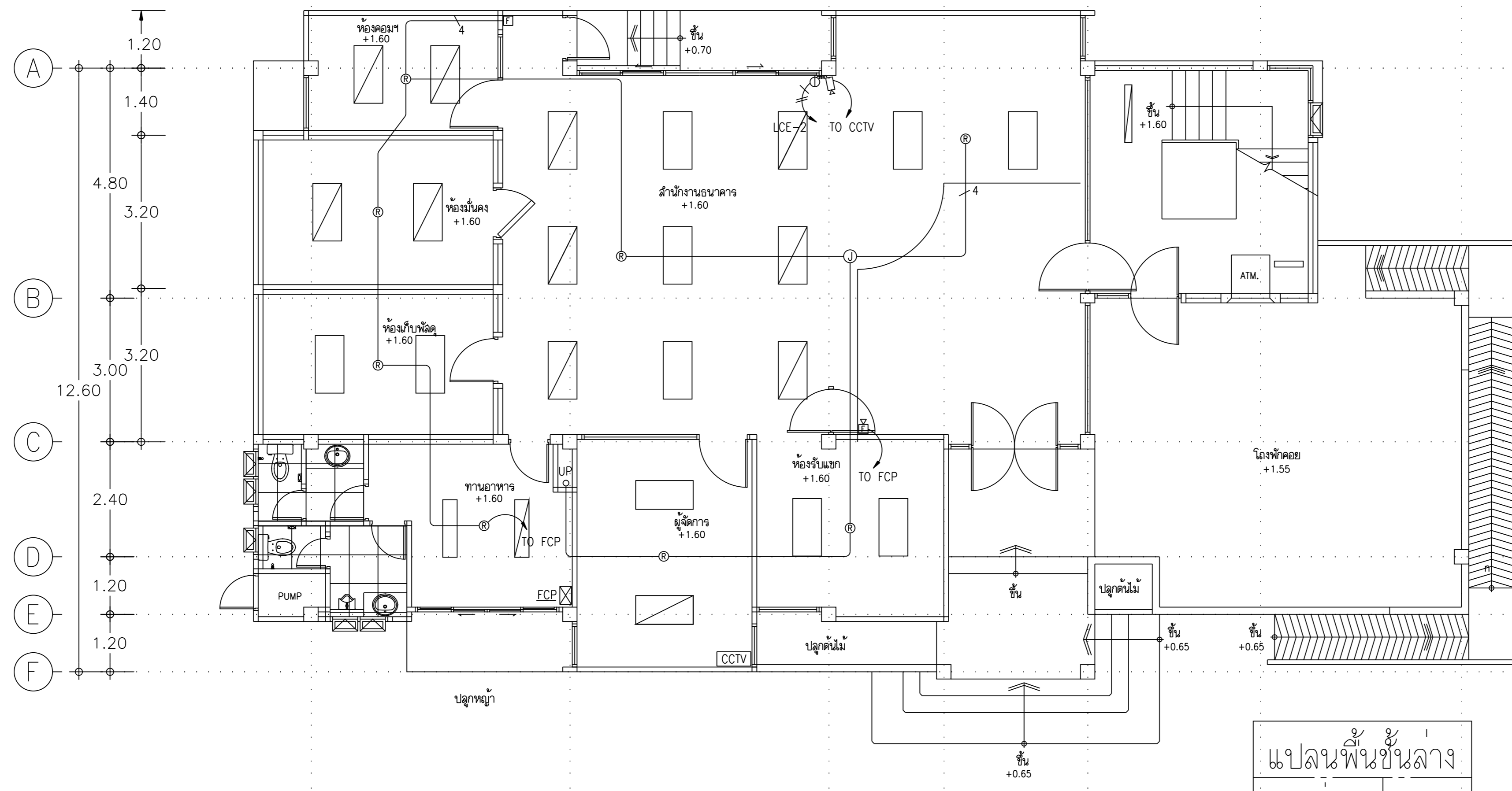
แปลนพื้นที่ชั้น 2 มาตราส่วน 1 : 100
